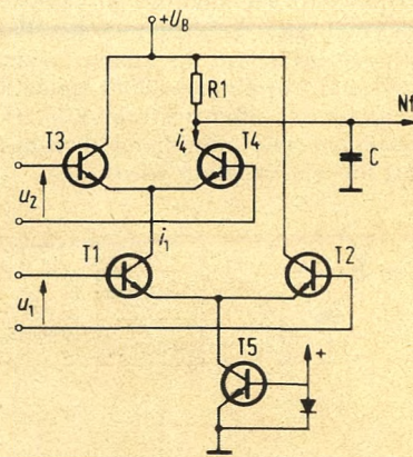
Bild 40. Prinzipschaltung eines Koinzidenzdemodulators innerhalb einer integrierten Schaltung (ULN 2111 von Sprague)
