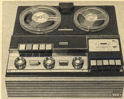
Kombiniertes Tonbandgerät für Band und Cassetten mit Überspielmöglichkeit von Band auf Cassette und umgekehrt (Aufnahme: Wiener Schwachstromwerke)
