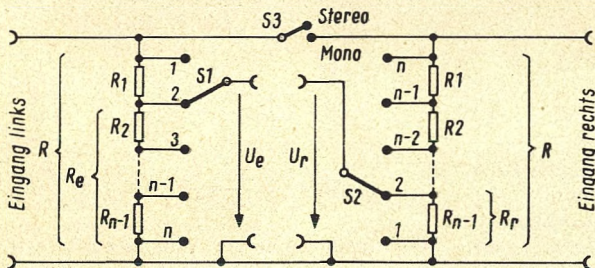
Bild 2. Richtungseinsteller für monaurale und stereofone Programme
