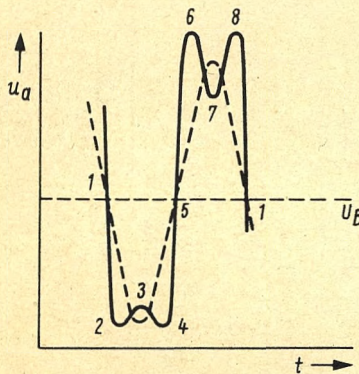
Bild 3. Zur Erläuterung der Wirkungsweise der Zusatzkreise in Bild 1 und 2 (nach Siemens-Halbleiter-Schaltbeispiele 1970)
