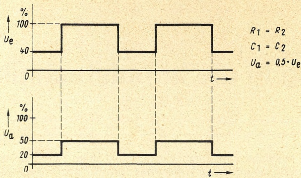
Bild 5.10. Ein frequenzunabhängiger Spannungsteiler verringert sowohl den Rechteckpuls als auch die überlagerte Gleichspannung
