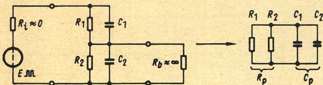
Bild 5.8. Frequenzkompensierter Spannungsteiler, Ersatzschaltbild zum Berechnen der Zeitkonstante
