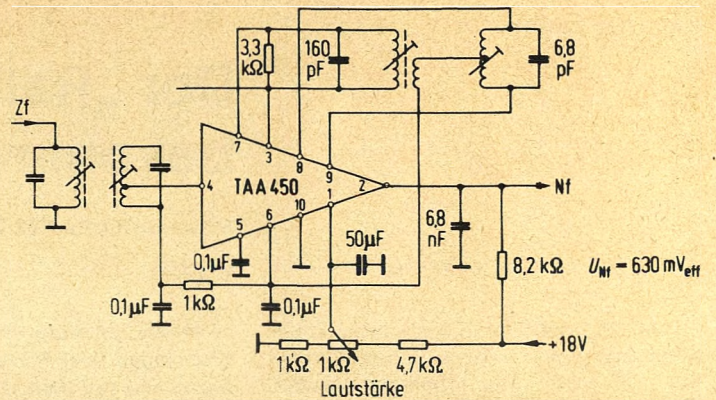
Bild 33. Ton-Zf-Verstärker, Ratiodektor und Nf-Verstärker mit der integrierten Schaltung TAA 450
