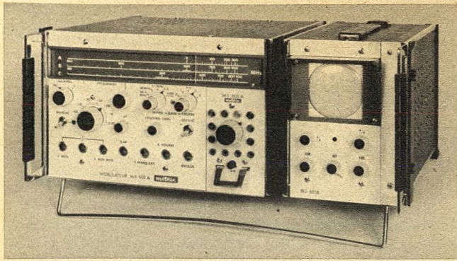
◀ Bild 2. Wobbler WX 601 A von Metrix mit angesetztem Sichtgerät
