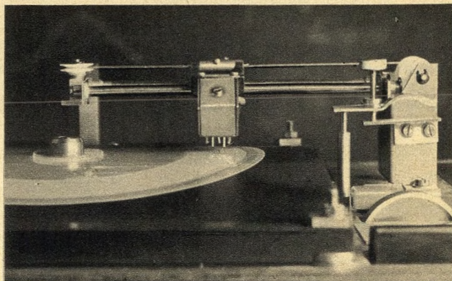
Bild 2. Auf diesem noch labormäßig gestalteten Plattenspieler wurde die Bildplatte in Berlin vorgeführt
