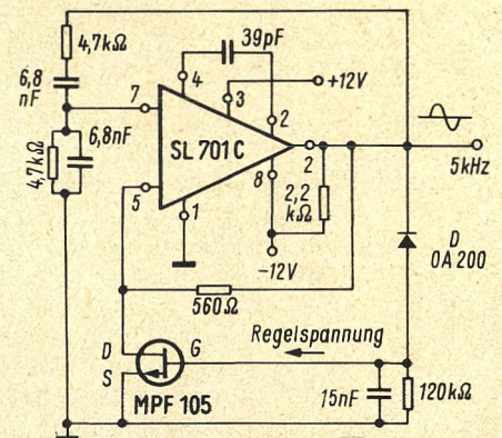
Schaltung eines Oszillators mit konstanter Amplitude durch eine Feldeffekttransistor-Regelschaltung. Die Regelung bewirkt zugleich eine bessere Frequenzkonstanz. Diese Wien-Brückenschaltung liefert eine Sinus-Ausgangsspannung von 5 kHz
