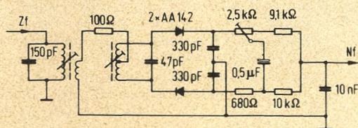
Bild 28. Ratiodektor nach Telefunken-Unterlagen
