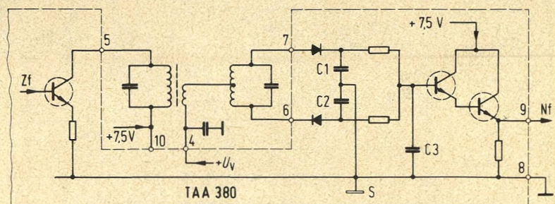
Bild 30. Demodulator und Nf-Verstärker in der integrierten Schaltung TAA 380 (gestrichelt umrandet). Das Ratiofilter ist außen anzuschließen
