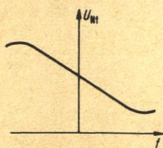
◀ Bild 38. Die Kennlinie eines Koinzidenzdemodulators verläuft ähnlich wie bei anderen FM-Detektoren
