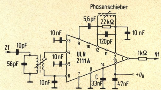
► Bild 44. Darstellung des Zf-Verstärkers innerhalb der Gesamtschaltung eines Empfängers (Telefunken)
