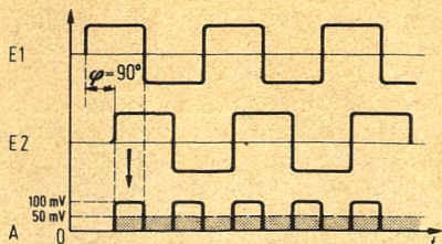
Bild 35. Impulsdarstellung der Funktion eines Koinzidenzdemodulators für eine Phasenverschiebung \varphi = 90^\circ
