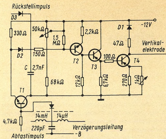
Bild 3. Die Schaltung zur Helligkeitssteuerung beim Matsushita-Schirm. An jedem der 230 Abgriffe der Verzögerungsleitung befindet sich diese Steuereinheit
