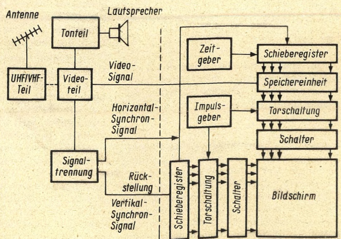
Bild 2. ▶ Empfängerschaltung mit Lumineszenzbildschirm und digitaler Steuerlogik von Mitsubishi
