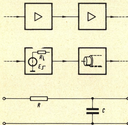
Bild 5.11. Galvanische Kopplung mit kapazitiver Last; Beispiele und Ersatzschaltbild
