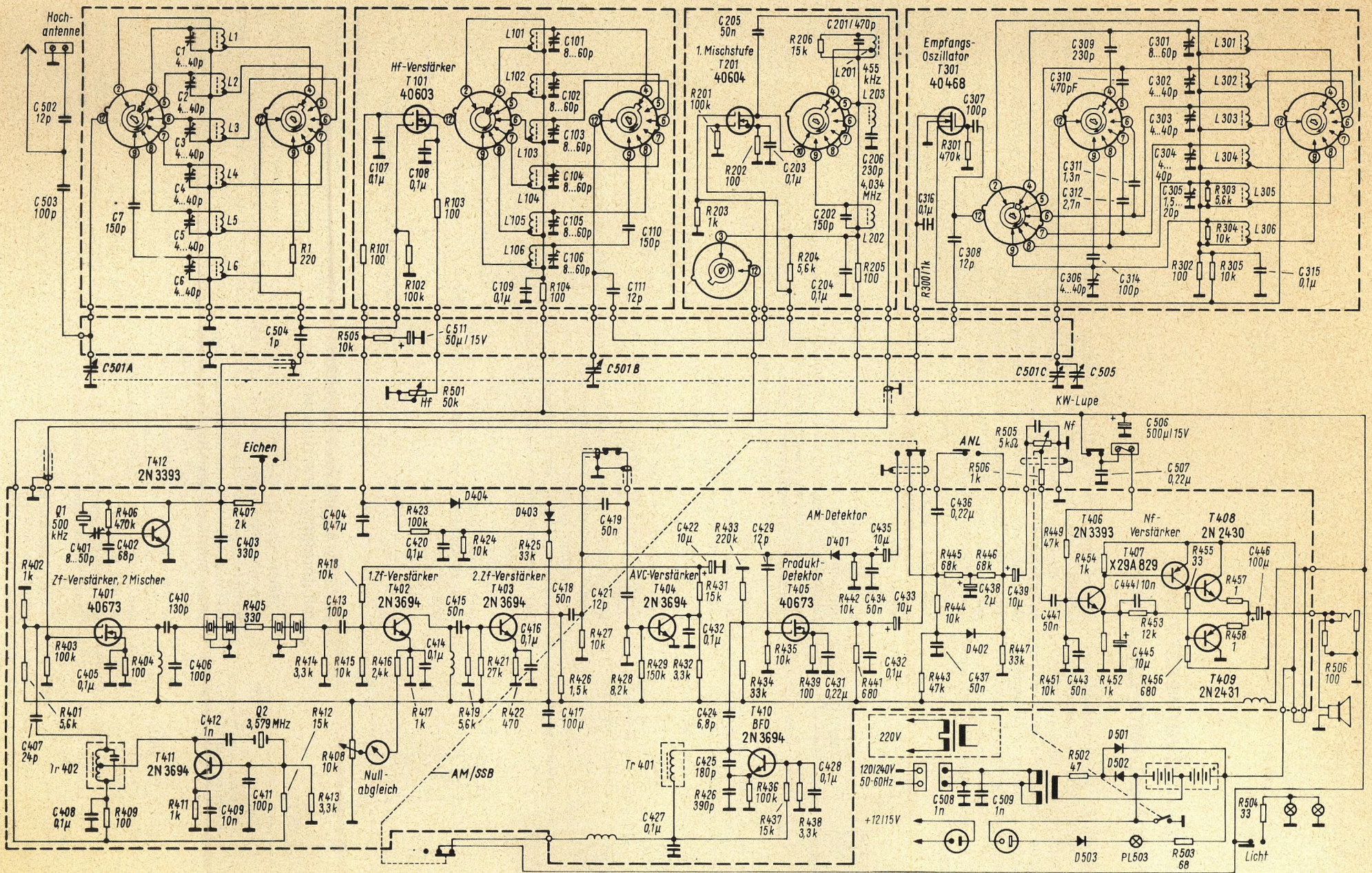
Bild 2. Die Gesamtschaltung des Gerätes
