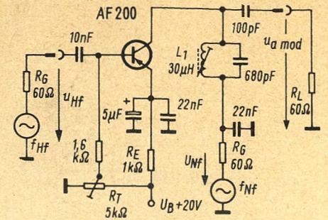
Einfache Modulationsschaltung mit geringem Klirrfaktor
