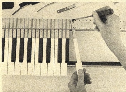
Bild 4. Montage eines Manuals
